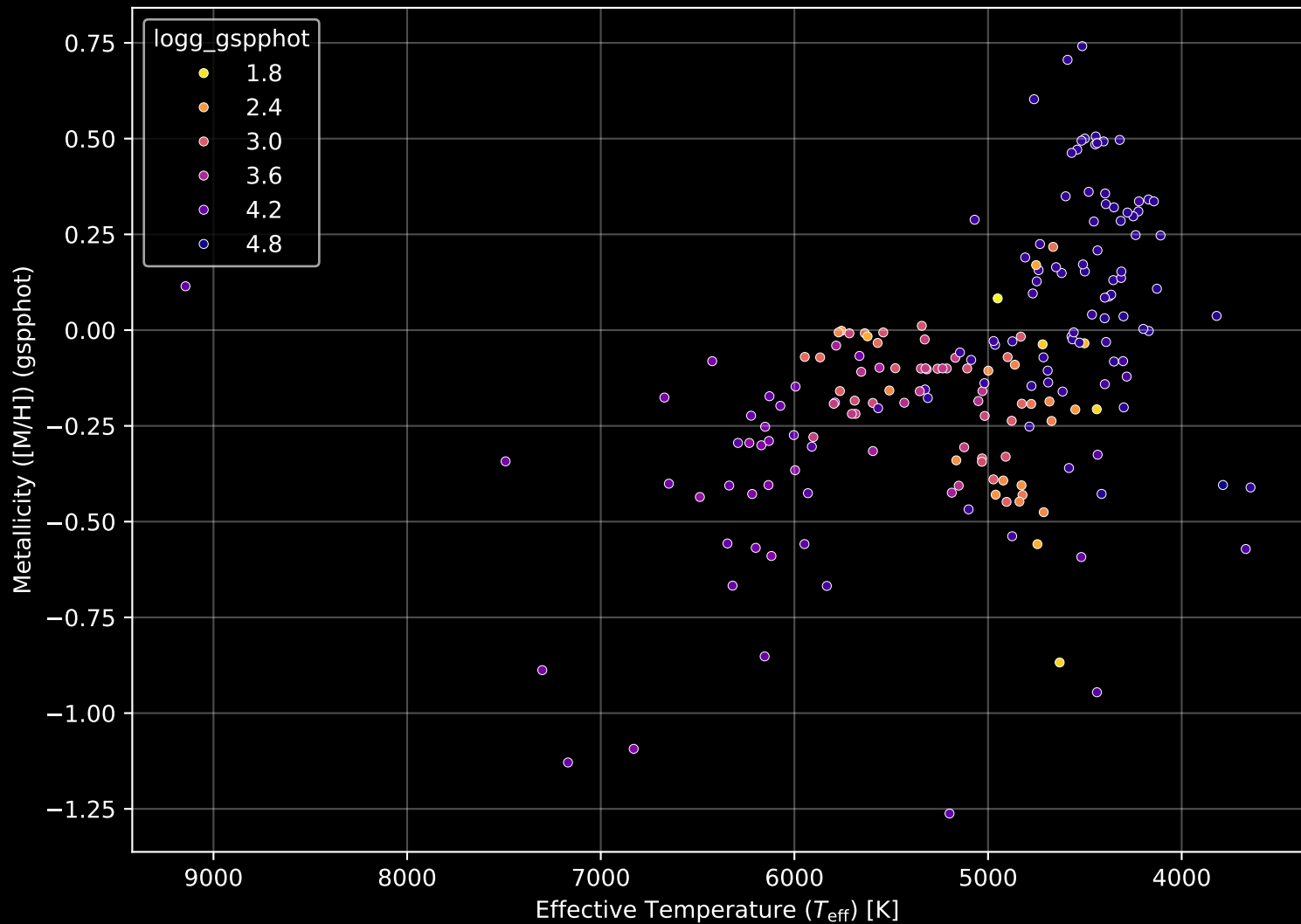
APOGEE DR17 Field: [279+66] Stellar Population Parameters (n= 191)
